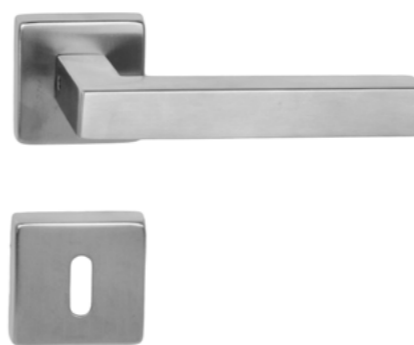
/// készleten CUBIC F szálciszított acél A rozsdamentes acél M A=130 mm D=50x50 mm
