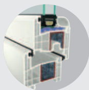
6 kamrás rendszer síkban eltolt szárny
