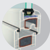
5 kamrás rendszer síkban eltolt szárny
